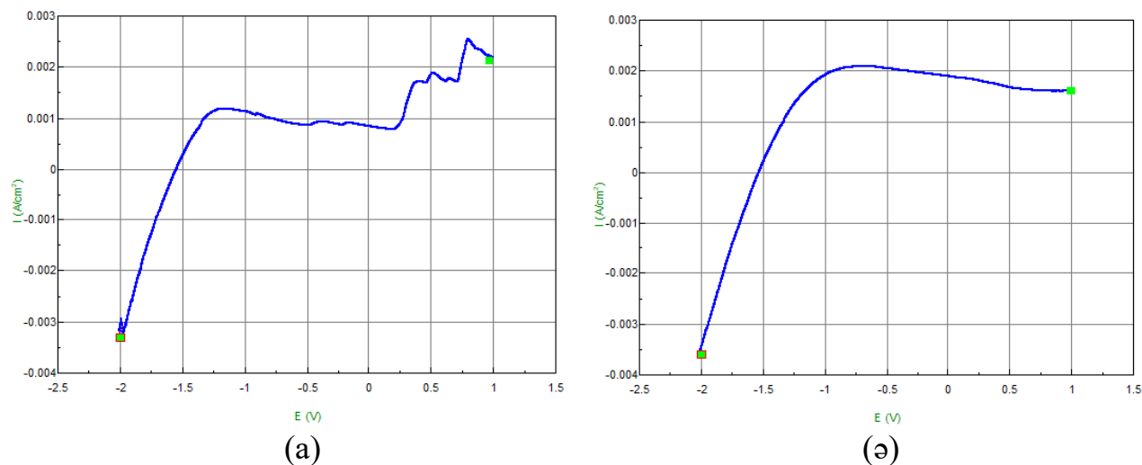
Сурет 4.8 – Алюминий электродының 0,1М NaOH ерітіндісіндегі анодтық вольтамперограммалары: а) потенциал беру жылдамдығы 100 мВ/с; ә) потенциал беру жылдамдығы 150 мВ/с
