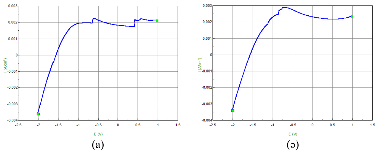
Сурет 4.9 – Алюминий электродының 0,1М NaOH ерітіндісіндегі анодтық вольтамперограммалары: а) потенциал беру жылдамдығы 200 мВ/с; ә) потенциал беру жылдамдығы 250 мВ/с
