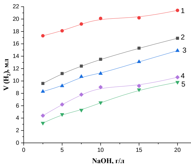
Сурет 3.38 – Алюминийдің әртүрлі құймаларының сілтілі ерітінділермен әрекеттесуі кезінде бөлінетін сутек көлемінің өзгеруі: 1 – Al-Mg; 2 – Al; 3 – дюралюминий; 4 – ЦАМ; 5 – силумин; S(\text{Al}) = 2,4 \text{ см}^2 , \tau = 5 минут
