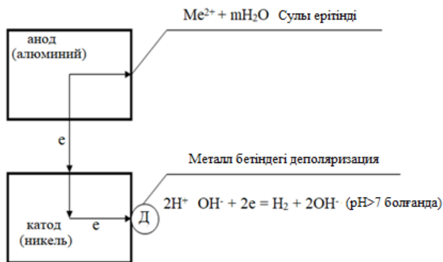
Сурет 5.2 – Алюминий және басқа металл арасында түзілген қысқа тұйықталған гальвани элементінің схемасы
