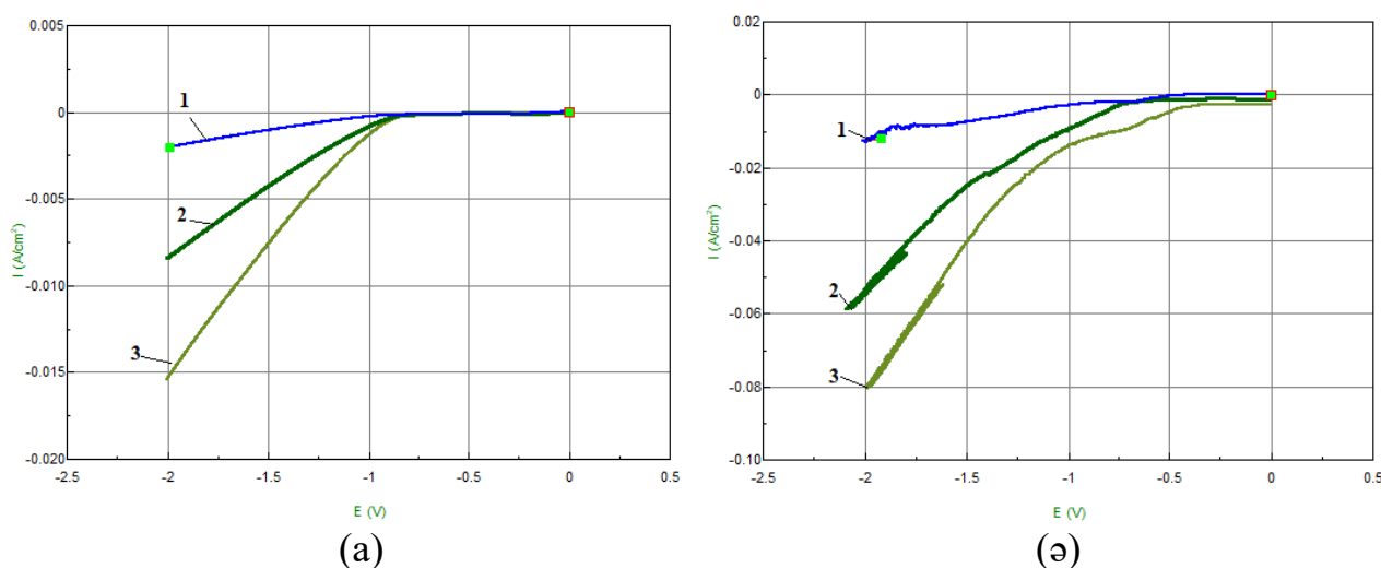
Сурет 4.6 – Платина электродында түсірілген катодтық потенциодинамикалық поляризациялық қисықтар, V = 50 мВ/с; t = 25^\circ\text{C} : а) 2 г/л \text{Hg}(\text{NO}_3)_2 ; 1 – 1,0 г/л \text{NaNO}_3 ; 2 – 5,0 г/л \text{NaNO}_3 ; 3 – 10,0 г/л \text{NaNO}_3 ; ә) 5,0 г/л \text{NaNO}_3 ; 1 – 1,0 г/л \text{Hg}(\text{NO}_3)_2 ; 2 – 5,0 г/л \text{Hg}(\text{NO}_3)_2 ; 3 – 10,0 г/л \text{Hg}(\text{NO}_3)_2 .
