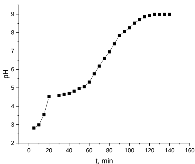
Сурет 3.5 – Судан сынап иондары қатысында алюминий электродында сутек бөліну барысында ерітінді \text{pH} -ның тәжірибе ұзақтығына байланысты өзгеруі: \text{C}(\text{Hg}(\text{NO}_3)_2) = 2 \text{ г/л} ; \tau = 140 \text{ мин.} ; \text{S}(\text{Al}) = 10 \text{ см}^2
