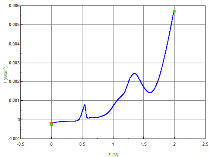
Сурет 4.7 – Құрамында сынап иондары бар натрий нитраты ерітіндісінде платина электродында түсірілген анодтық поляризациялық қисық: t = 25^{\circ}\text{C} , V = 50 \text{ мВ/с} ; 1,0 \text{ г/л NaNO}_3 ; 2,0 \text{ г/л Hg (NO}_3)_2
