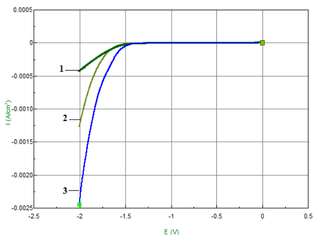
Сурет 4.1 – Алюминий электродының натрий нитраты ерітіндісінде түсірілген катодтық поляризациялық қисықтары, \text{NaNO}_3 , г/л: 1 – 1,0; 2 – 5,0; 3 – 10,0; t = 25^\circ ; V = 50 \text{ мВ/с}
