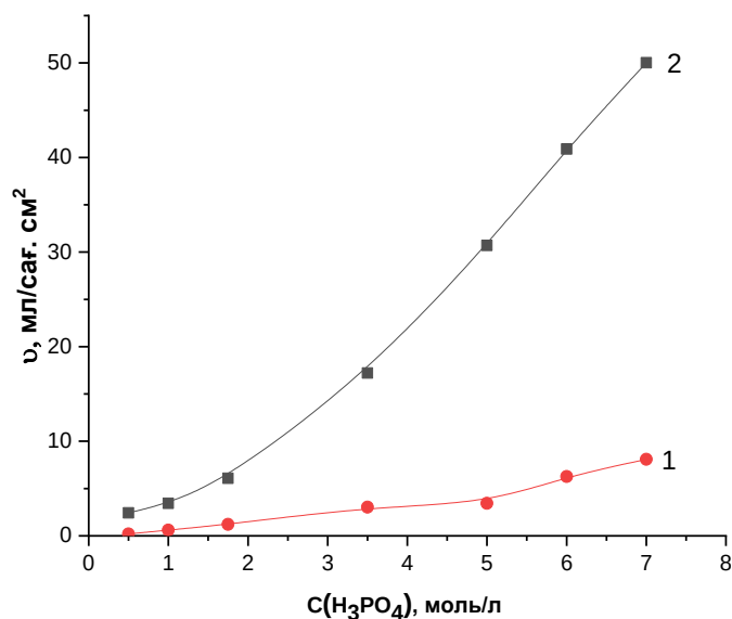
Сурет 3.34 – Алюминий электродының фосфор қышқылымен әрекеттесуі кезінде сутек газының бөліну жылдамдығына қышқыл концентрациясының әсері: \tau = 0,06 сағ., S(Al) = 8,23 см 2 : 1 – тек фосфор қышқылымен әрекеттескенде; 2 – фосфор қышқылына 25 г/л NaCl қосқан кезде
