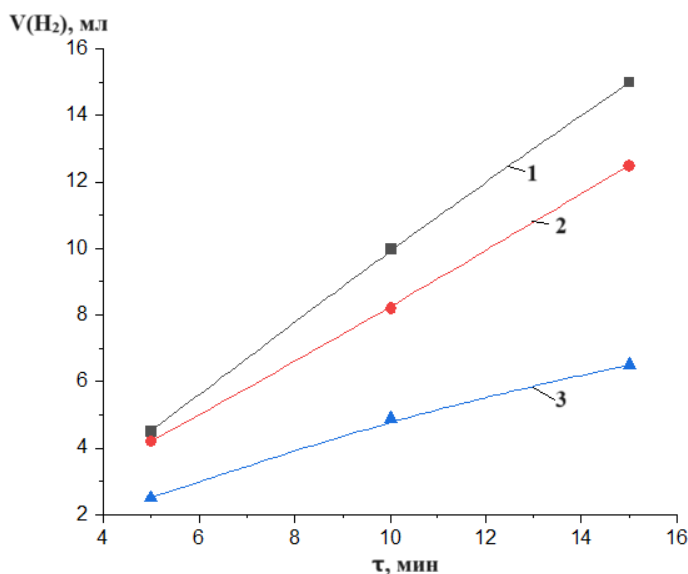
Сурет 3.29 – Судан сутек бөліну көлеміне су құрамының әсері: \text{Hg}(\text{NO}_3)_2 – 0,1 г/л, t = 25^\circ\text{C} . 1 – құбыр суы, 2 – дистилденген су, 3 – дист.су + 0,5 г/л NaCl
