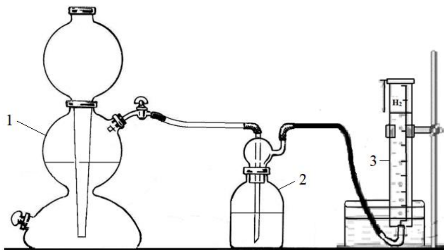
Сурет 2.3 – Сынап (II) тұзы (нитраты) қатысында алюминийдің сумен әрекеттесуі кезінде бөлінетін сутек газын тазартуға арналған қондырғы. Мұнда:
