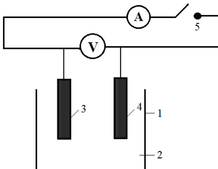
Сурет 2.4 – Алюминий және бірқатар металдармен құрылған гальваникалық жұптардағы электр қозғаушы күш пен қысқа тұйықталған токты өлшеуге арналған қондырғының принципиалды схемасы: 1 – электролизер; 2 – электролит; 3 – алюминий электроды; 4 – екінші электрод; V – жоғары омдық вольтметр; A – амперметр; 5 – кілт
