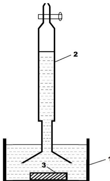
Сурет 2.2 – Лабораторияда сутек алу үшін жиналған қондырғы 1 – су құйылған кең ыдыс; 2 – шкаласы бар шыныдан жасалған бюретка; 3 – алюминий электроды (пластинасы)
