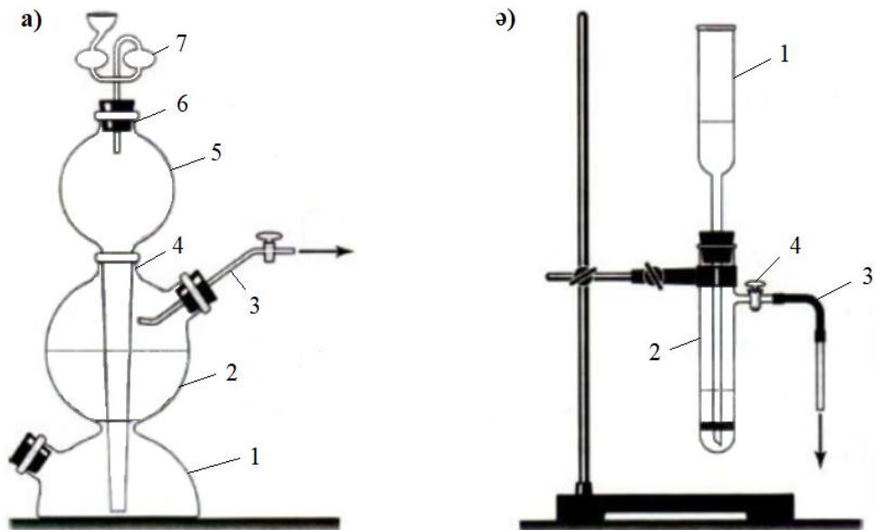
Сурет 2.1 – Лабораторияда сутек алу үшін қолданылатын қондырғылар: а) Кипп аппараты, мұнда 1 – резервуар; 2 – газ шығаруға арналған түтігі бар колба – реактор; 3 – газ шығаратын тубус (түтік); 4 – колба-реактордың мойыны; 5 – груша тәріздес воронка; 6 – воронканың мойыны; 7 – сақтандырғыш воронка; ә) Кирюшкин аспабы, мұнда: 1 – воронка; 2 – пробирка; 3 – шыныдан жасалған шланг; 4 – кран (зажим)
