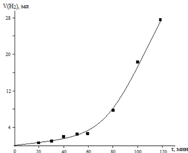
Сурет 3.10 – Алюминий мен суды катализатор қатысында (3,0 г/л) әрекеттестіру кезінде бөлінетін сутектің көлемінің тәжірибе ұзақтығына байланысты өзгеруі, t = 30^{\circ}\text{C} ; S(\text{Al}_{\text{пл.}}) = 24 \text{ см}^2
