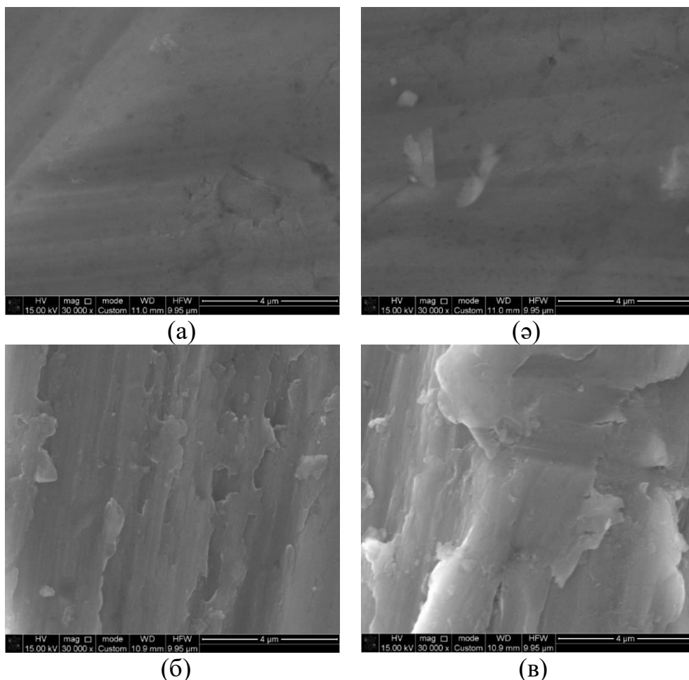
Сурет 3.36 – Алюминий электродының беттік қабатының 30 000 есе үлкейтілген СЭМ фотосуреті
