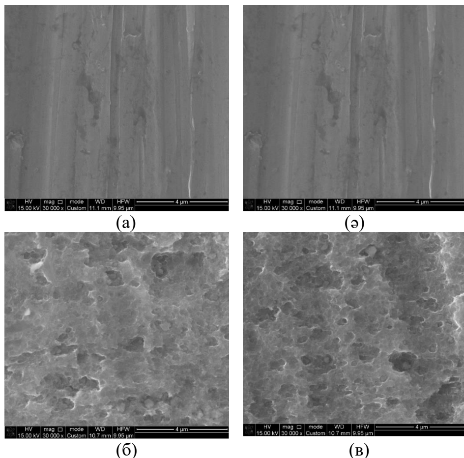
Сурет 3.19 – Алюминий электродының беттік қабатының 30 000 есе үлкейтілген СЭМ фотосуреттері: а, ә – дистильденген суға батырылғаннан кейін кептірілген күйі; б,в – натрий гидроксидінің ерітіндісіне батырылғаннан кейін кептірілген күйі
