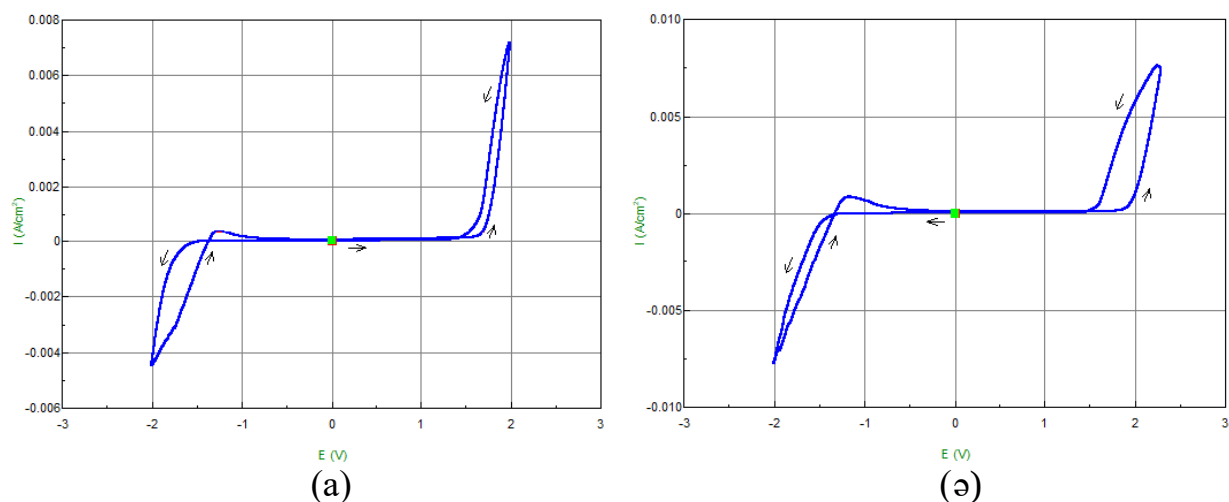
Сурет 4.4 – Алюминий электродының \text{NaNO}_3 - 50,0\text{ г/л} ; V = 50\text{ мВ/с} ; t = 25^{\circ}\text{C} болғанда түсірілген циклді потенциодинамикалық поляризациялық қисықтары: а) анодтық-катодтық; ә) катодтық-анодтық
