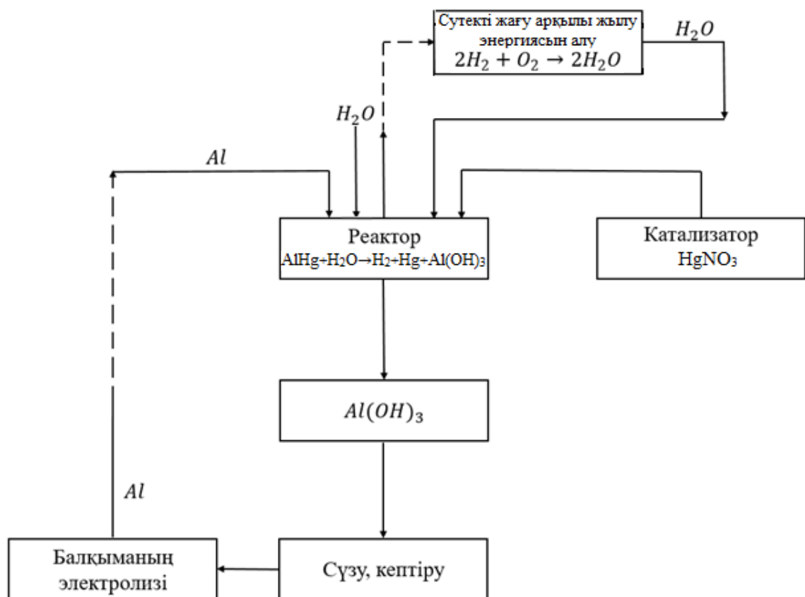
Сурет 3.17 – Су мен алюминийді катализатор қатысында әрекеттестіріп сутек алу технологиясының принципиалды схемасы
