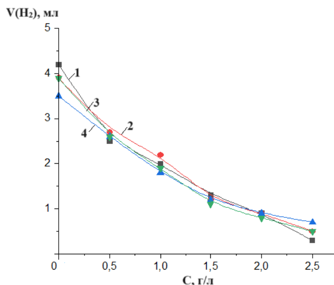
Сурет 3.25 – Металл катиондарының судан сутек бөліну жылдамдығына әсері (катализатор қатысында), Hg(NO_3)_2 - 0,1 г/л, \tau = 5 мин, t = 25^\circ C : 1 – NaCl, 2 – KCl, 3 – BaCl 2 , 4 – MgCl 2
