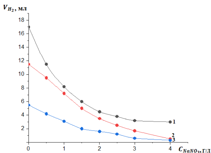
Сурет 3.22 – Сулы-сілтілі ерітіндіден сутек газының бөлінетін көлеміне натрий нитратының уақытқа байланысты әсері, S(\text{Al}_{\text{пл}}) = 16 \text{ см}^2 , 1 – 10 мин., 2 – 5 мин., 3 – 3 мин.
