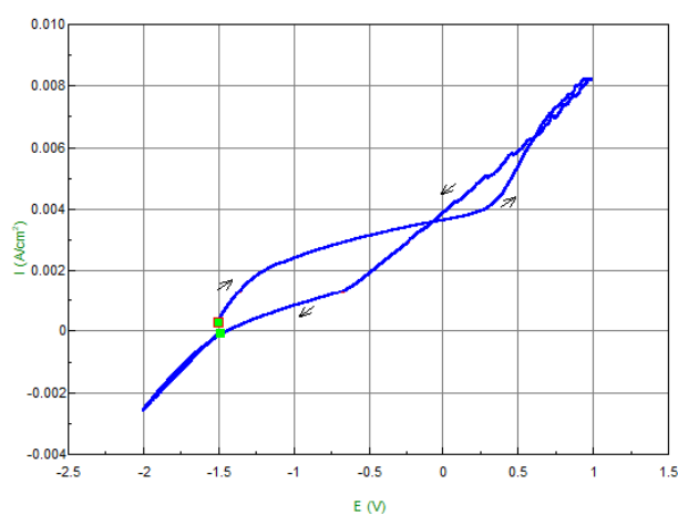
Сурет 4.11 – Алюминий электродының 0,1М NaOH ерітіндісіндегі анодтық-катодтық циклді вольтамперограммалары: а) потенциал беру жылдамдығы 100 мВ/с; ә) потенциал беру жылдамдығы 200 мВ/с;
