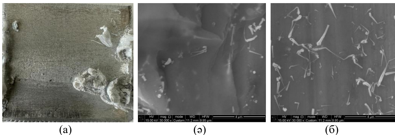
Сурет 3.37 – Судан сутек алу үшін пайдаланылатын алюминий электродының күкірт қышқылына натрий хлориді қосылған ерітіндіге батырылғаннан кейінгі фотосуреті (а); 30 000 есе үлкейтілген СЭМ фотосуреттері (э және б)
