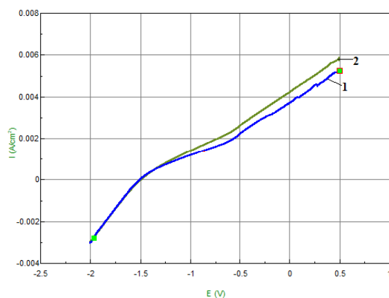
Сурет 4.10 - Алюминий электродының 0,1М NaOH ерітіндісіндегі катодтық вольтамперограммалары: 1 – потенциал беру жылдамдығы 100 мВ/с; 2 – потенциал беру жылдамдығы 200 мВ/с
