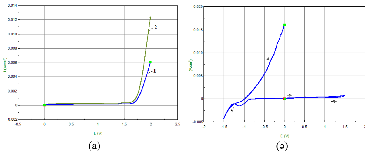
Сурет 4.5 – Құрамында сынап иондары бар натрий нитраты ерітіндісінде түсірілген поляризациялық қисықтар, V = 200 мВ/с; t = 25^\circ\text{C} болғанда: а) анодтық: 1 – 50,0 г/л \text{NaNO}_3 ; 2 – 50,0 г/л \text{NaNO}_3 + 1,0 г/л \text{Hg}(\text{NO}_3)_2 ; ә) циклді анодтық-катодтық: 50,0 г/л \text{NaNO}_3 + 1,0 г/л \text{Hg}(\text{NO}_3)_2
