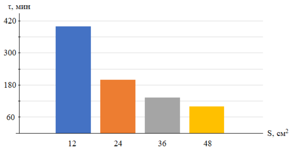
Сурет 3.11 – Көлемі 25 мл сутек бөліну үшін қажет болатын уақыттың ( \tau ) өзгеруіне алюминийдің беттік ауданының ( S ) әсері, 1,0 г/л катализатор қатысында
