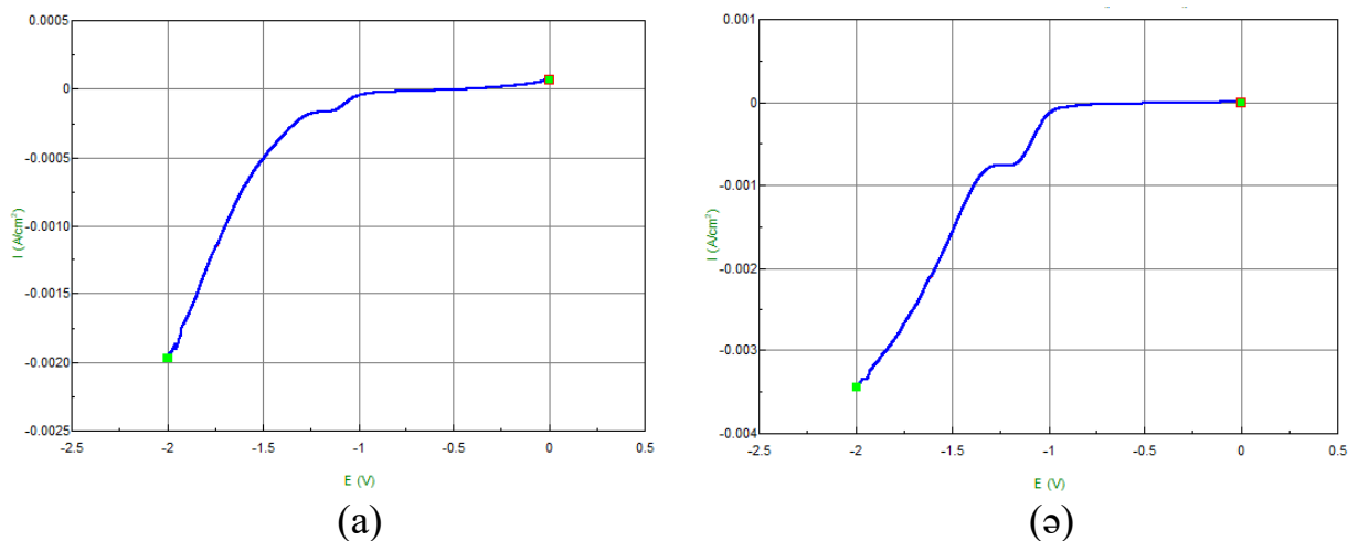
Сурет 4.2 – Құрамында сынап иондары бар 5,0 г/л натрий нитраты ерітіндісінде, t = 25^{\circ}\text{C} , V = 50 мВ/с-ке тең болғанда алюминий электродында түсірілген катодтық поляризациялық қисықтар: а) 0,5 г/л \text{Hg}(\text{NO}_3)_2 ; ә) 1,0 г/л \text{Hg}(\text{NO}_3)_2
