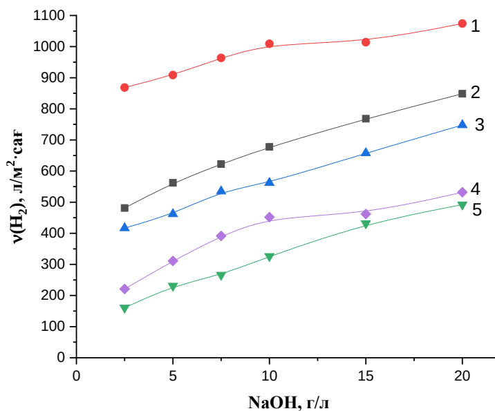
3.39 сурет – Алюминийдің әртүрлі құймаларының сілтілі ерітінділермен әрекеттесуі кезінде сутек бөліну жылдамдығының өзгеруі: 1 – Al-Mg; 2 – Al; 3 – дюралюминий; 4 – ЦАМ; 5 – силумин; S(\text{Al}) = 2,4 \text{ см}^2 , \tau = 5 минут
