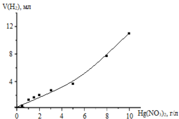
Сурет 3.9 – Катализатор концентрациясының бір сағатта бөлінетін сутек газының көлеміне әсері, t = 30^{\circ}\text{C} , S(\text{Al}) = 24 \text{см}^2
