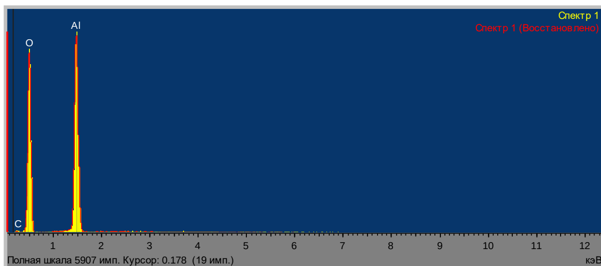
Сурет 3.12 – Судан катализатор қатысында сутек алу реакциясынан кейін түсірілген алюминий пластинасының бетінің рентгенофлуоресценттік спектрі
