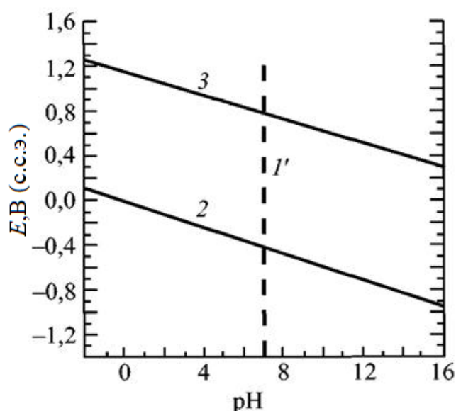
Сурет 3.1 – Судың E-pH диаграммасы (t = 25°C)
