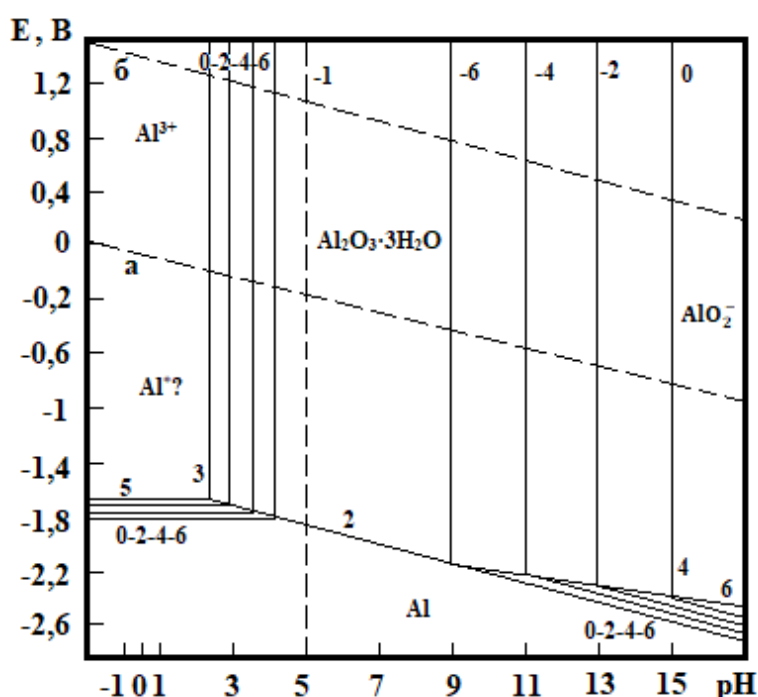
Сурет 3.3 – Алюминий мен судан құрылған жүйедегі Е-рН диаграмма
