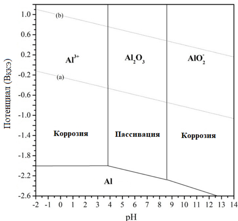
Сурет 3.2 – Al-H 2 O жүйесінің E-pH диаграммасы (t=25°C)
