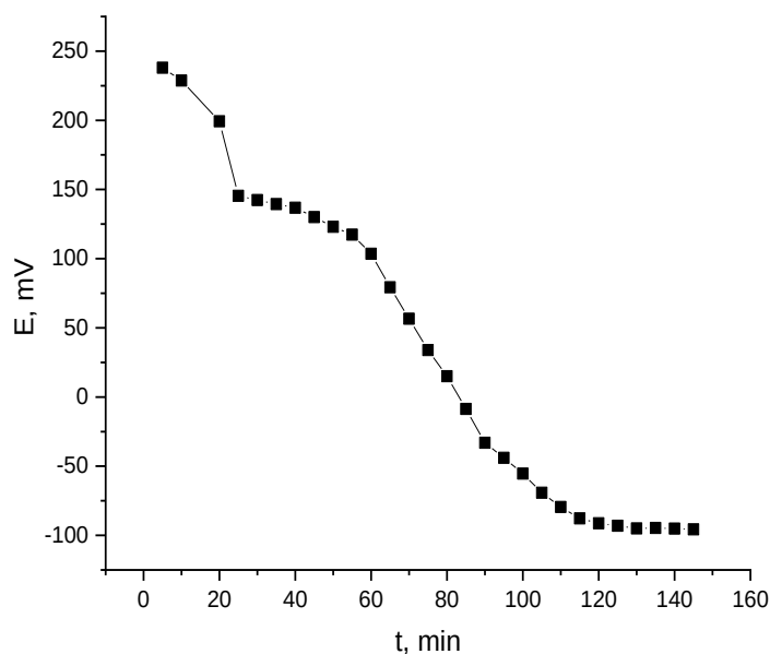
Сурет 3.6 – Судан сынап иондары қатысында алюминий электродында сутек бөліну барысында потенциалдың тәжірибе ұзақтығына байланысты өзгеруі: C(\text{Hg}(\text{NO}_3)_2) = 2 \text{ г/л}; = 2 \text{ г/л}; \tau = 140 \text{ мин.}; S(\text{Al}) = 10 \text{ см}^2
