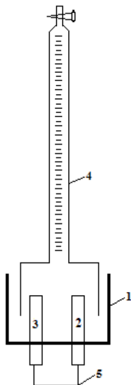
Сурет 5.1 – Судан сутек алу үшін жиналған қондырғының принципиялды схемасы: 1 – ерітінді құйып, электродтар орналастыратын стакан, 2 – алюминий электроды; 3 – екінші қосалқы электрод; 4 – реакция барысында бөлінетін сутек көлемін өлшеуге арналған бюретка; 5 – электр өткізгіш сым
