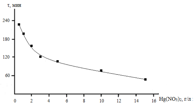
Сурет 3.8 – Көлемі 25 мл-ге сутек бөліну үшін қажет болатын уақыттың ( \tau ) катализатор концентрациясына тәуелділігі ( t = 30^{\circ}\text{C} ), S(\text{Al}) = 24 \text{см}^2
