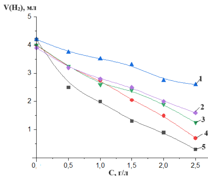
Сурет 3.28 – Аниондардың судан бөлінетін сутек көлеміне әсері (катализатор қатысында), \text{Hg}(\text{NO}_3)_2 – 0,1 г/л, \tau = 5 мин, t = 25^\circ\text{C} : 1 – \text{NaHCO}_3 , 2 – \text{NaNO}_3 , 3 – \text{NaNO}_2 , 4 – \text{Na}_2\text{SO}_4 , 5 – \text{NaCl}
