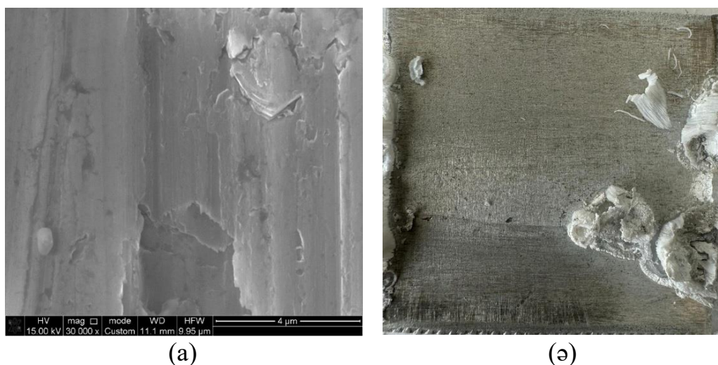
Сурет 3.32 – Алюминий электродының беттік қабатының СЭМ фотосуреті 30 000 есе үлкейтілген, а, ә – сынап нитратының ерітіндісіне батырылғаннан кейін кептірілген күйі
