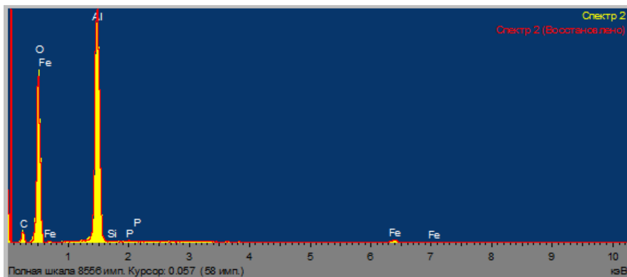
Сурет 3.15 – Судан сутек бөліну нәтижесінде түзілген тұнбаның энергиядисперсиялық рентгенофлуоресценттік спектрі
