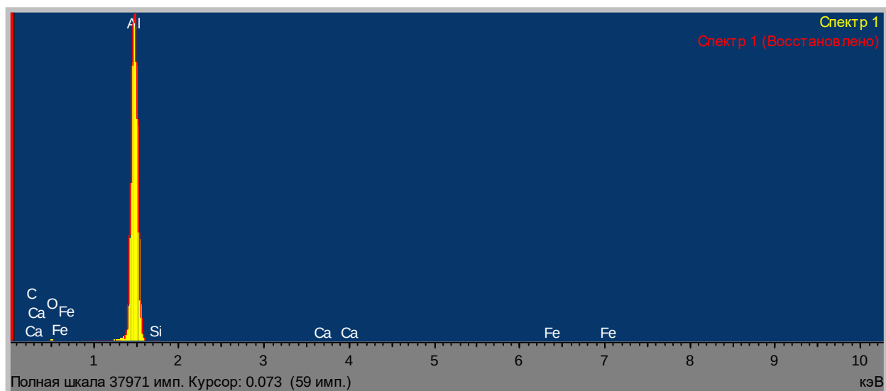
Сурет 2.6 – Судан сутек алу үшін қолданылатын алюминий электродының бастапқы күйдегі рентгенофлуоресценттік спектрі.
