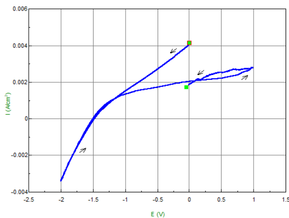
Сурет 4.12 – Алюминий электродының 0,1М NaOH ерітіндісіндегі катодтық-анодтық циклді вольтамперограммалары: а) потенциал беру жылдамдығы 100 мВ/с; ә) потенциал беру жылдамдығы 200 мВ/с
