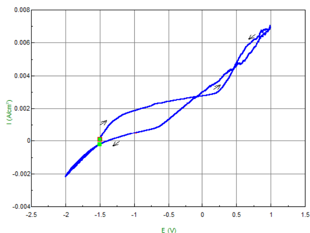
Сурет 4.11 – Алюминий электродының 0,1М NaOH ерітіндісіндегі анодтық-катодтық циклді вольтамперограммалары: а) потенциал беру жылдамдығы 100 мВ/с; ә) потенциал беру жылдамдығы 200 мВ/с;
