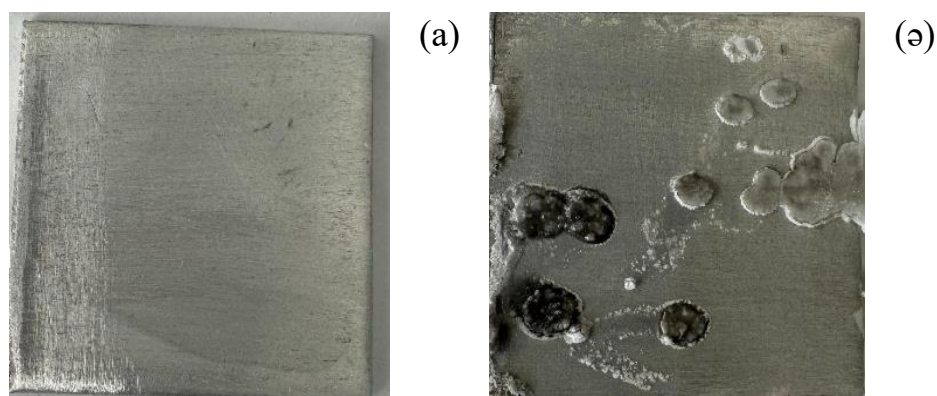
Сурет 3.35 – Судан сутек алу үшін пайдаланылатын алюминий пластинасының фотосуреті: а – фосфор қышқылының ерітіндісіне батырылғаннан кейінгі; ә – фосфор қышқылына натрий хлоридін қосқандағы ерітіндіге батырылғаннан кейінгі
