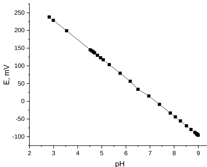
Сурет 3.4 – Судан сынап (II)иондары қатысында алюминий электродында сутек бөліну барысында ерітінді рН-ның потенциал мәніне байланысты өзгеруі:
