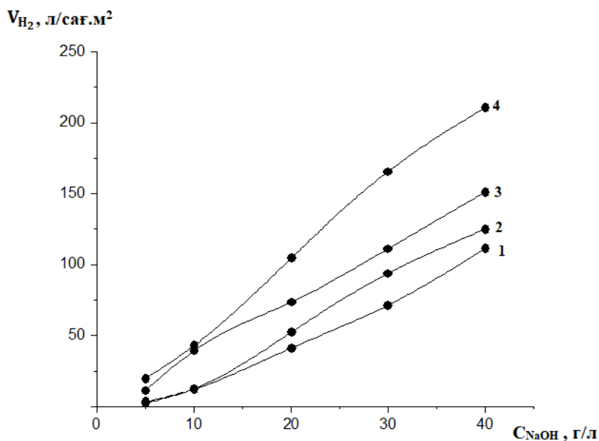
Сурет 3.18 – Алюминийдің сулы-сілтілі ерітінділермен әрекеттескенде сілті концентрациясының және алюминий пластинасының беттік ауданының сутек бөліну жылдамдығына әсері: S(Al): 1 – 1 см², 2 – 4 см², 3 – 9 см², 4 – 16 см²
