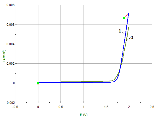
Сурет 4.3 – Алюминий электродының натрий нитраты ерітіндісіндегі әртүрлі потенциал беру жылдамдықтарында, t = 25^{\circ}\text{C} ; 50,0\text{ г/л NaNO}_3 болғанда түсірілген анодтық поляризациялық қисықтары: 1 – 10\text{ мВ/с} ; 2 – 200\text{ мВ/с} ;
