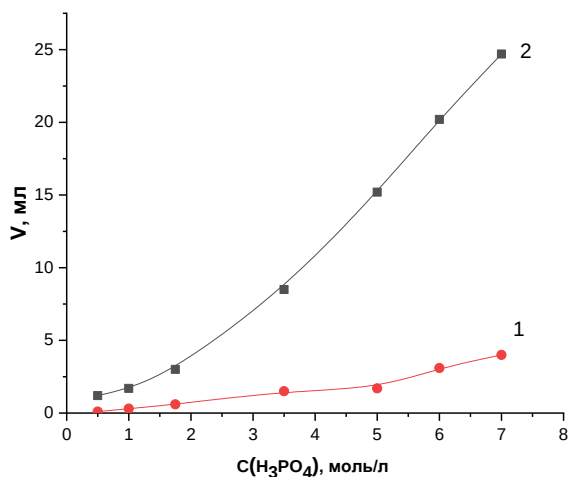
Сурет 3.33 – Алюминий электродының фосфор қышқылымен әрекеттесуі кезінде бөлінетін сутек көлеміне қышқыл концентрациясының әсері: \tau = 0,06 сағ., S(Al) = 8,23 см 2 : 1 – тек фосфор қышқылымен әрекеттескенде; 2 – фосфор қышқылына 25 г/л NaCl қосқан кезде
