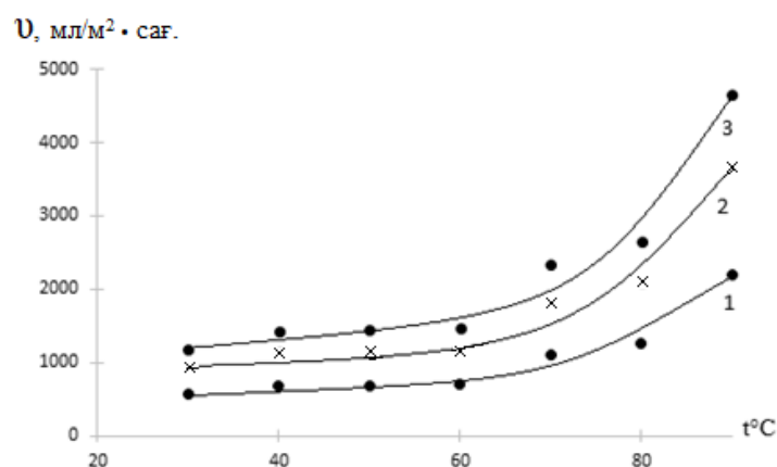
Сурет 3.7 – Сутек бөліну жылдамдығының катализатордың әртүрлі концентрациясында: 1 – 1 г/л; 2 – 2 г/л; 3 – 3 г/л температураға тәуелді түрде өзгеруі, \tau=1 сағ.; S=24 \text{см}^2
